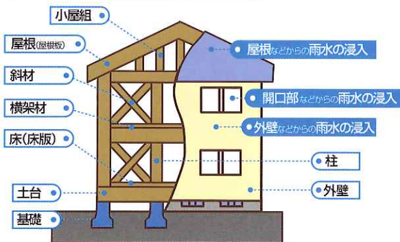
木造(在来軸組工法)の戸建住宅例
